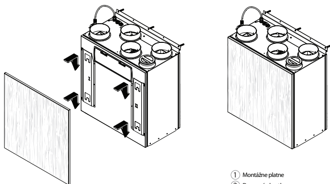
Obr. 13. Inštalácia nábytkovej dosky
