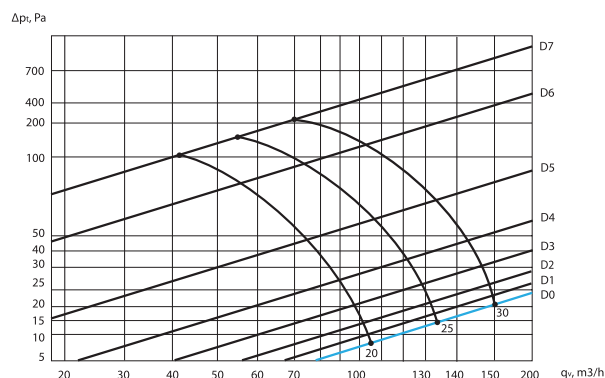
RONDO 150 (odvod vzduchu)
