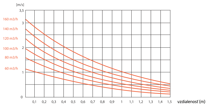
RONDO 150 rýchlosť, m/s
