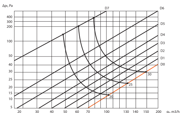
RONDO 150 (prívod vzduchu)
